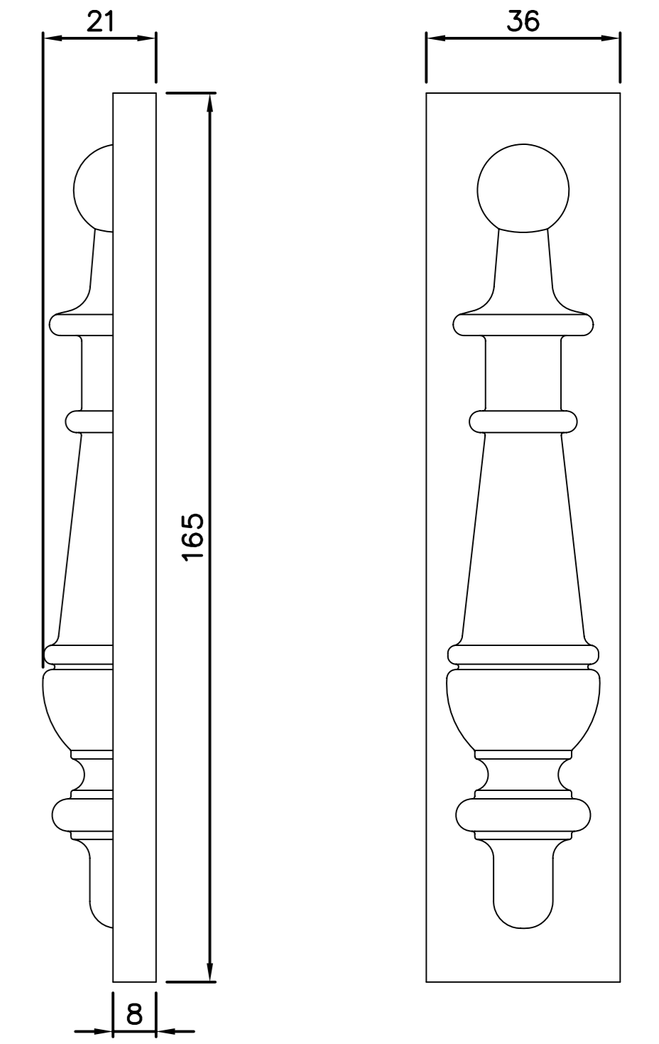
FG210 Zierstück
