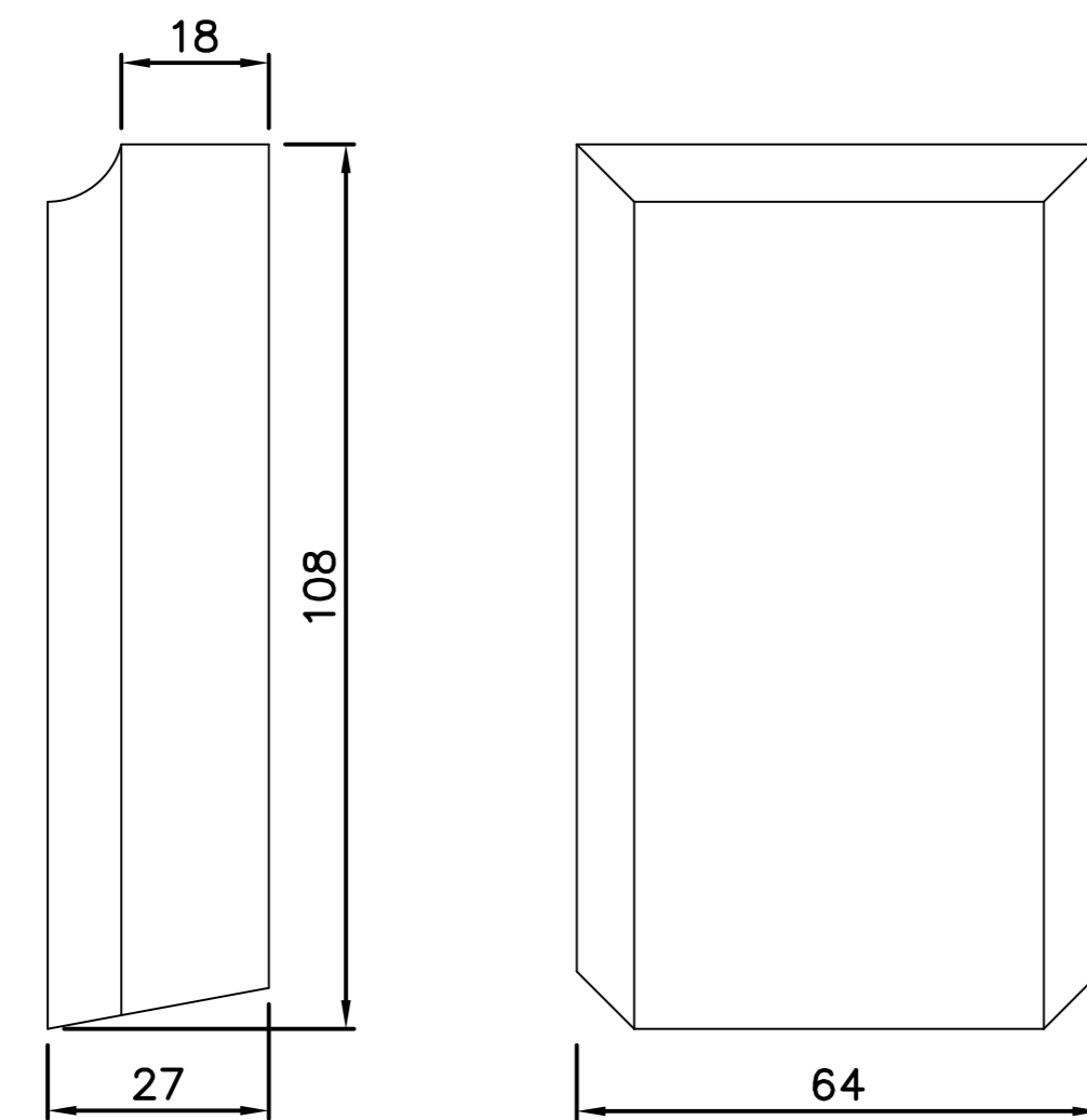
FG354 Zierstück
