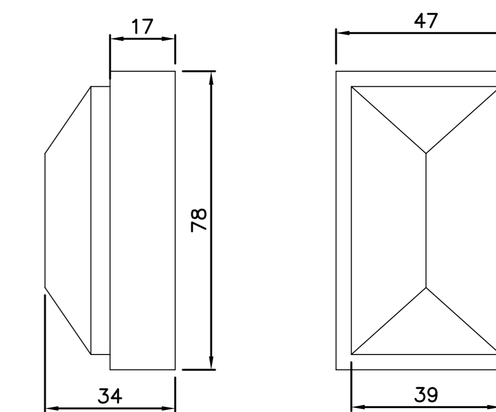
FG272 Zierstück
