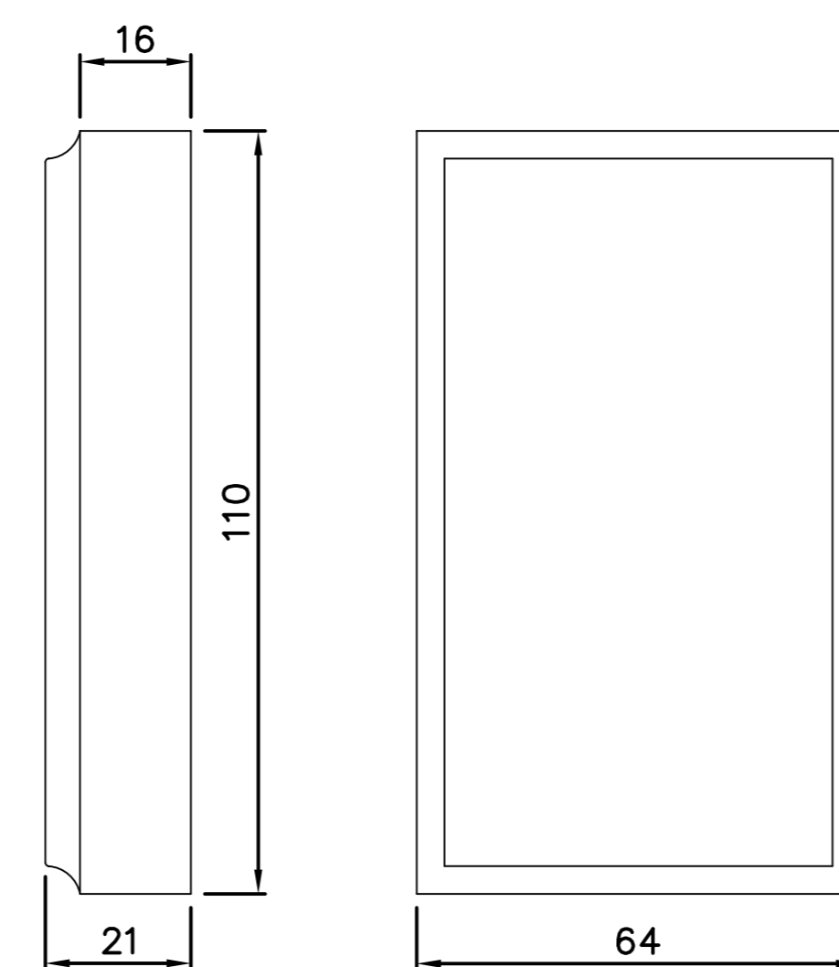
FG305 Zierstück
