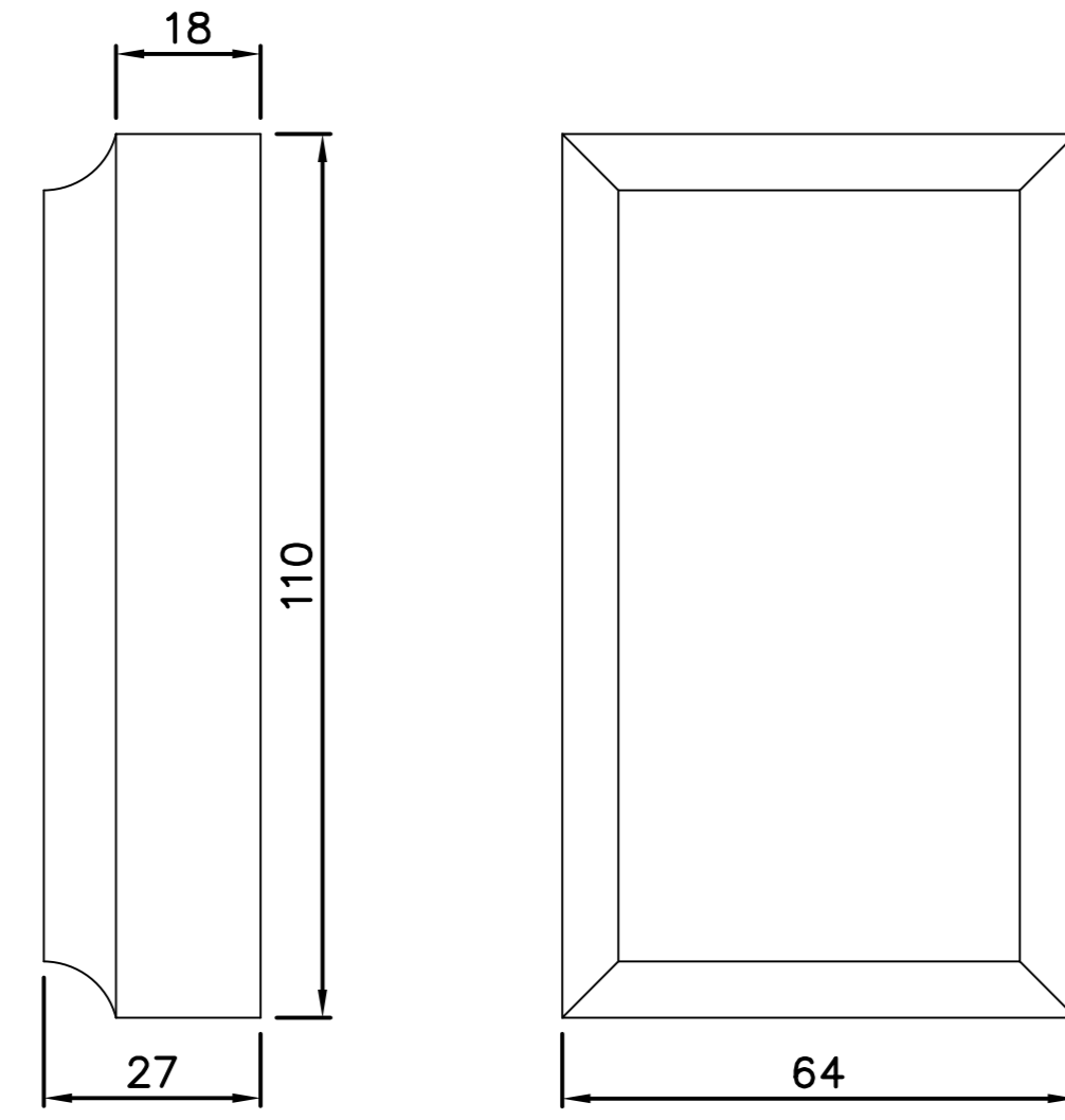
FG304 Zierstück
