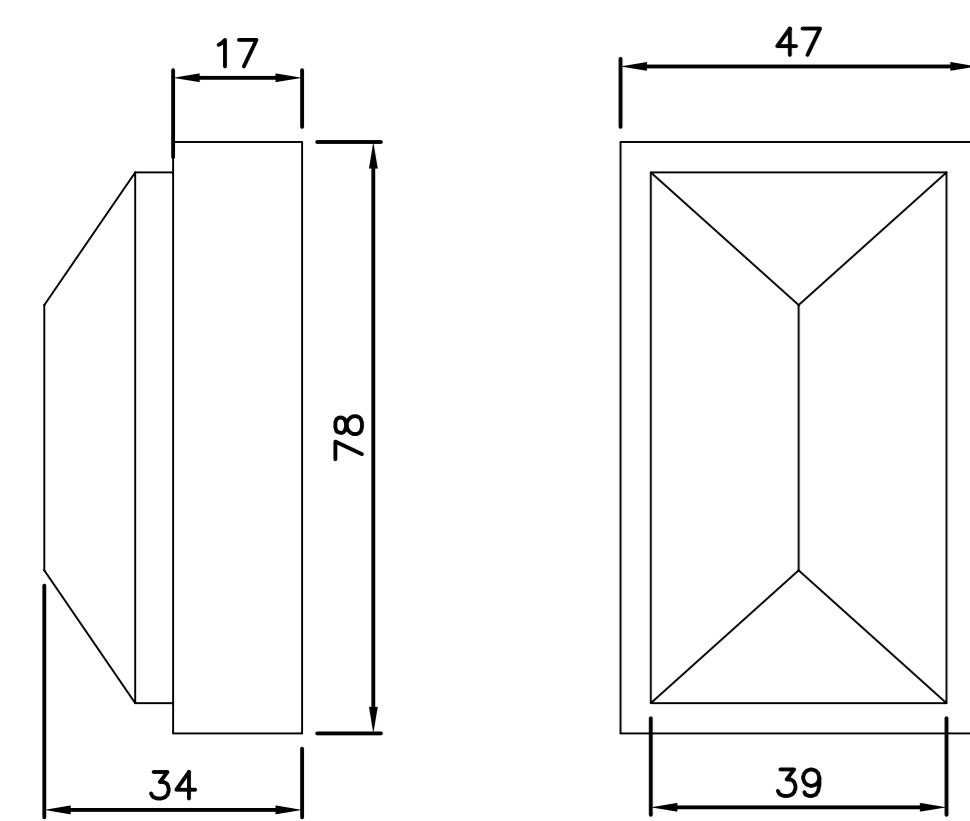
FG272 Zierstück
