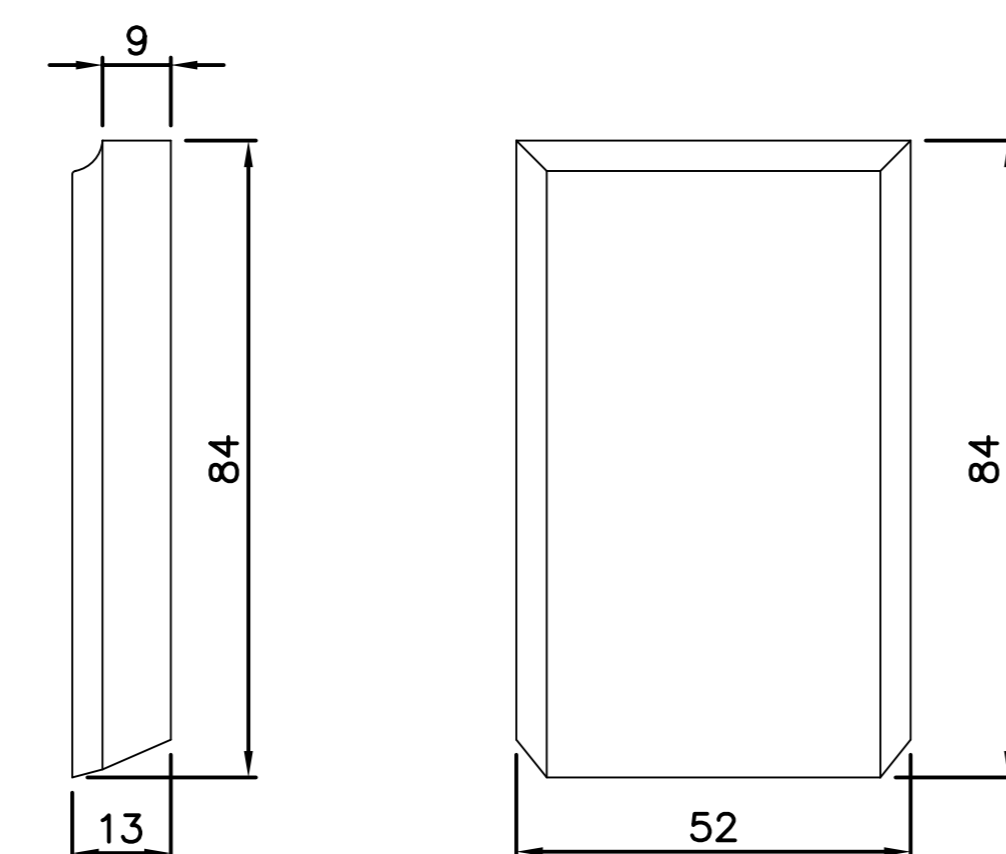
FG355 Zierstück
