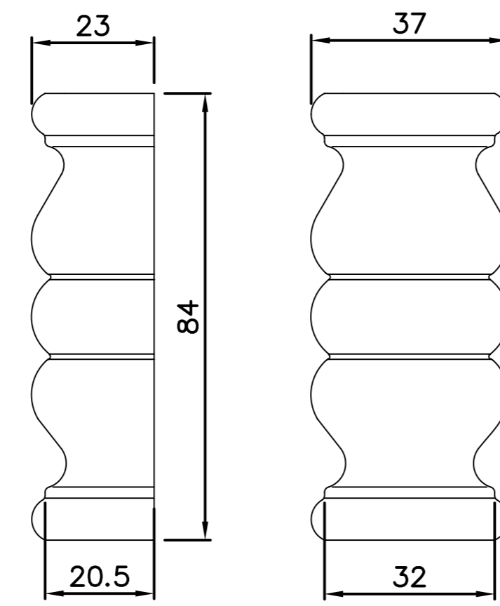
FG206 Zierstück
