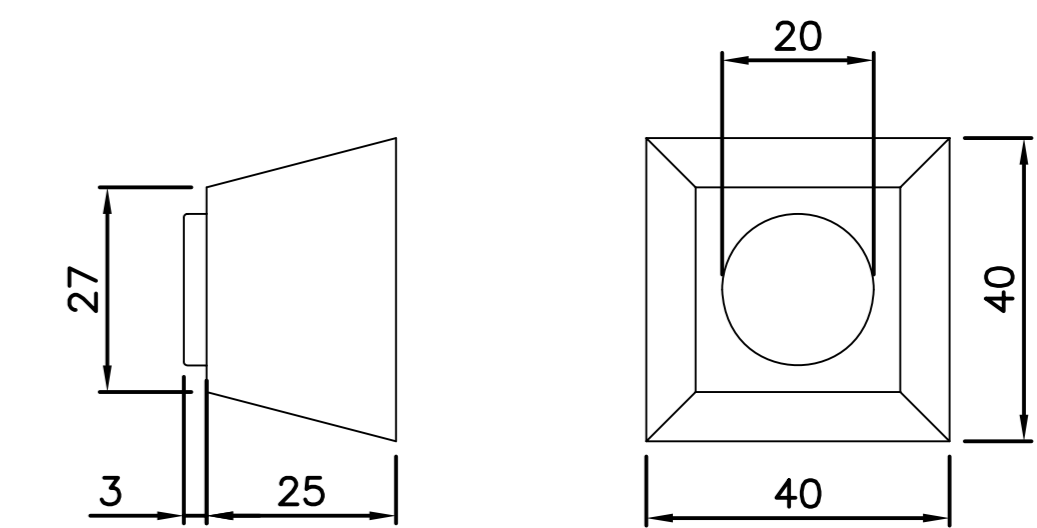
FG256 Zierstück
