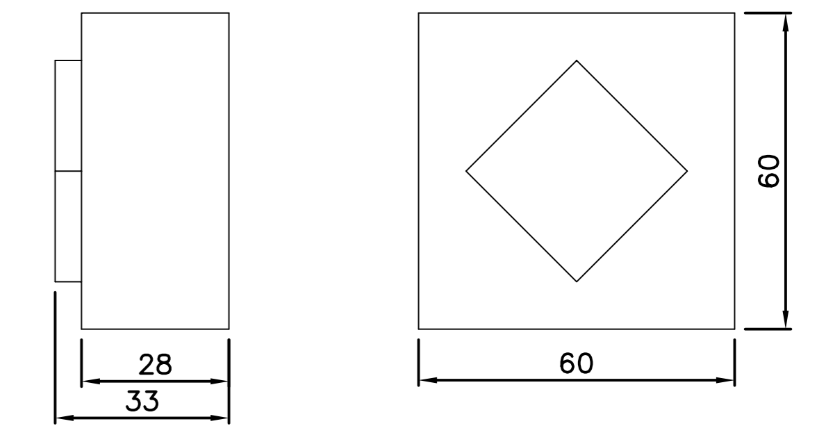
FG271 Zierstück
