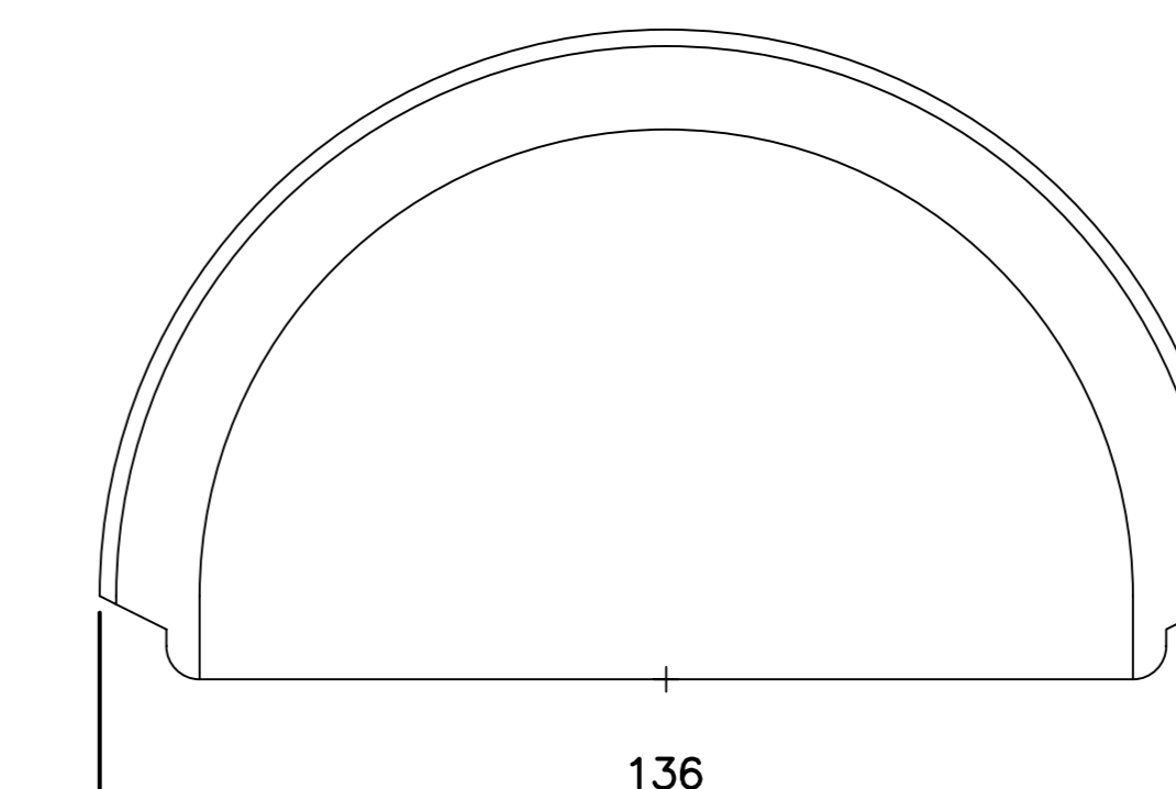
FG137 Zierstück
