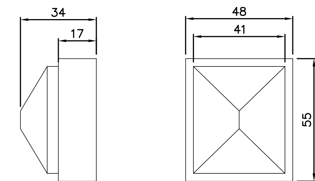
FG273 Zierstück
