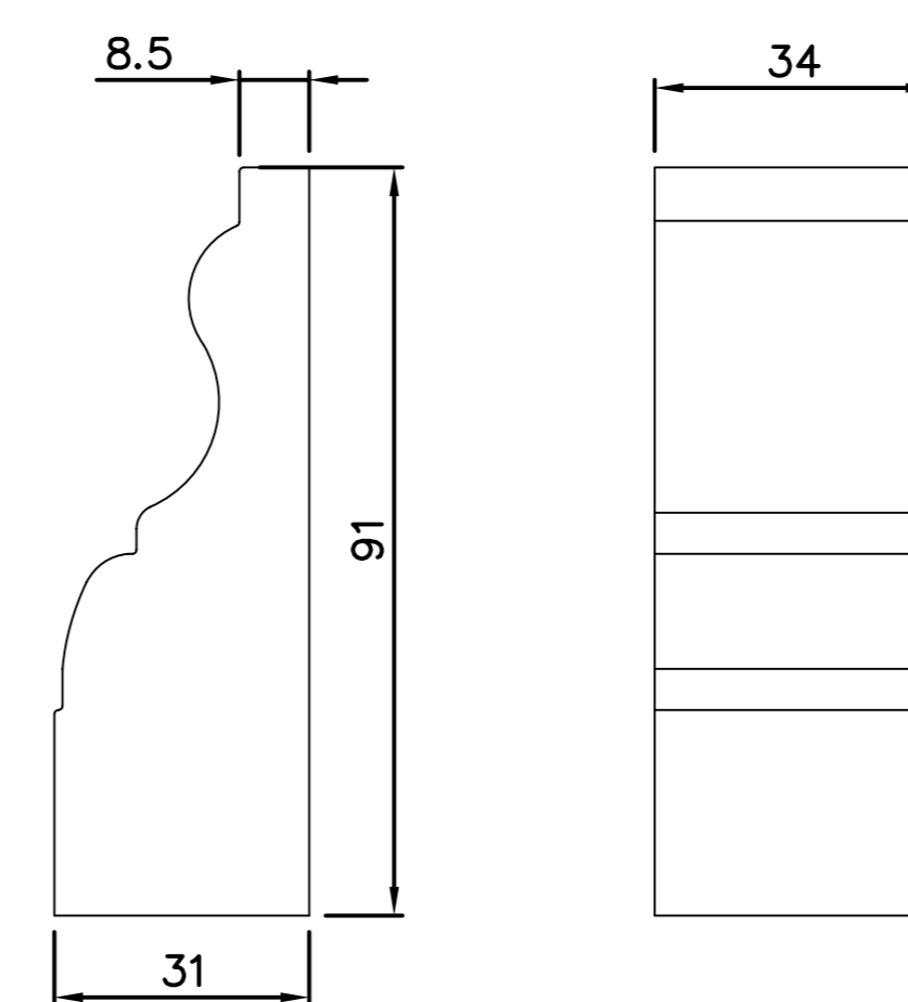
FG260 Zierstück
