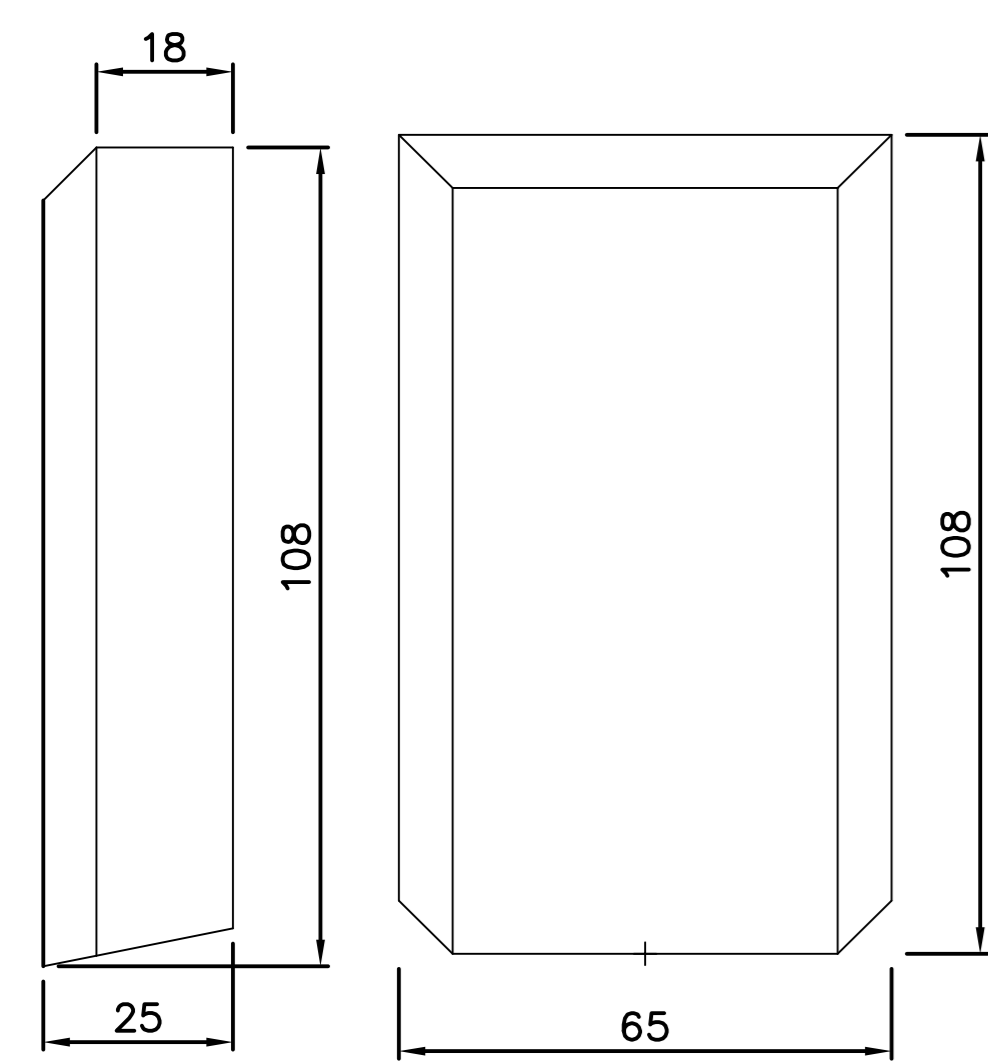
FG352 Zierstück
