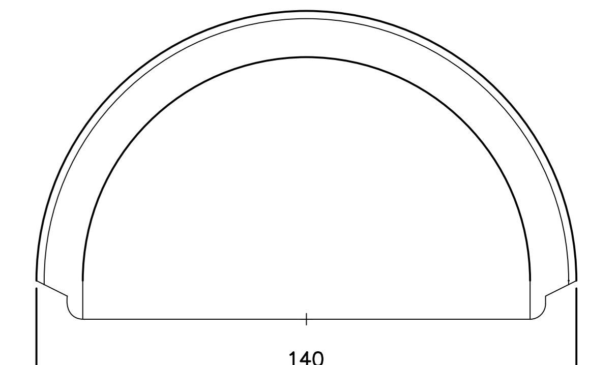
FG140 Zierstück
