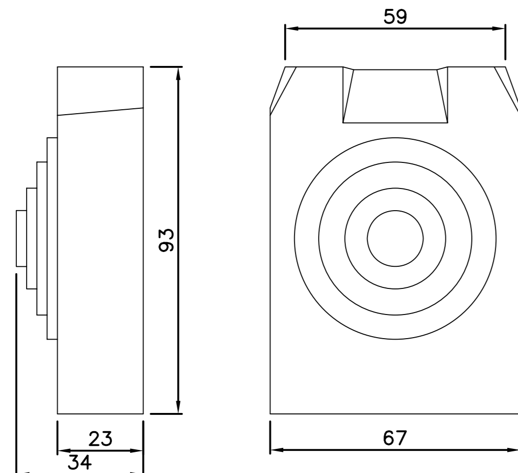
FG258 Zierstück
