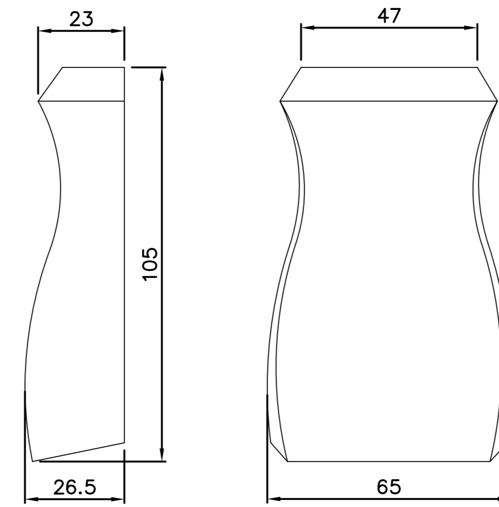
FG252 Zierstück
