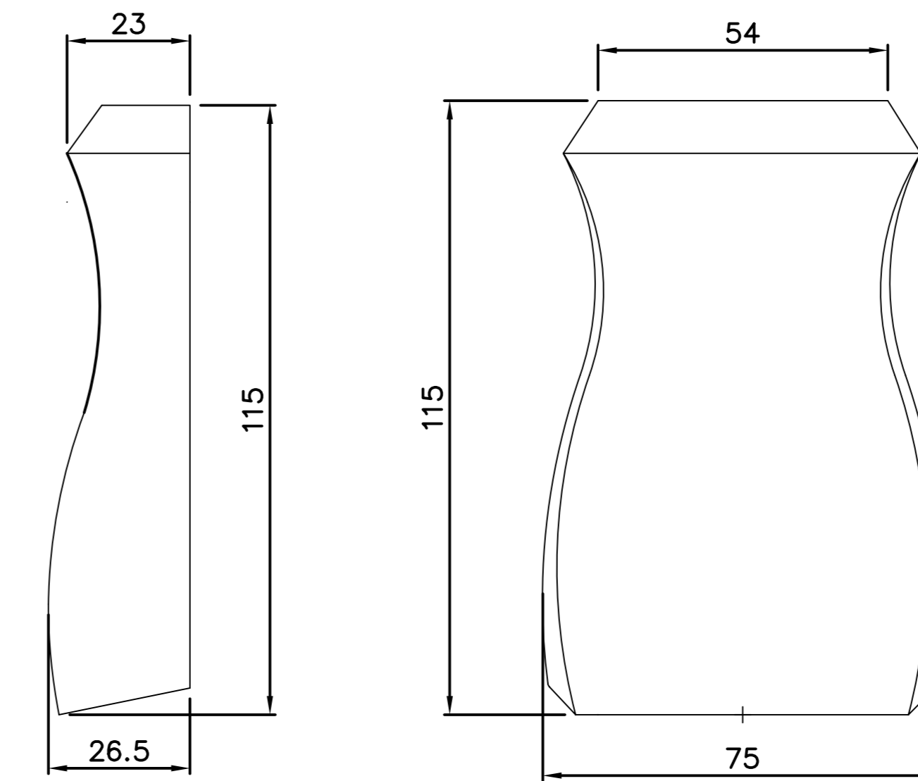
FG253 Zierstück
