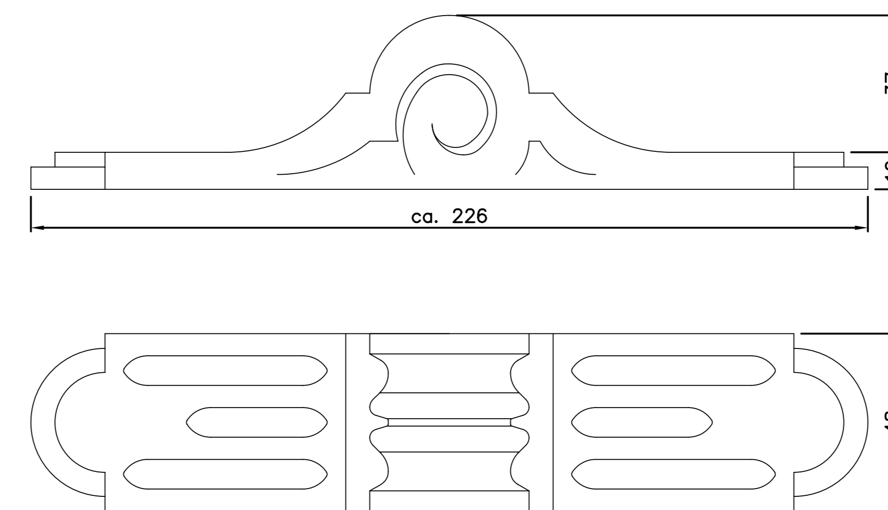
FG401 Zierstück
