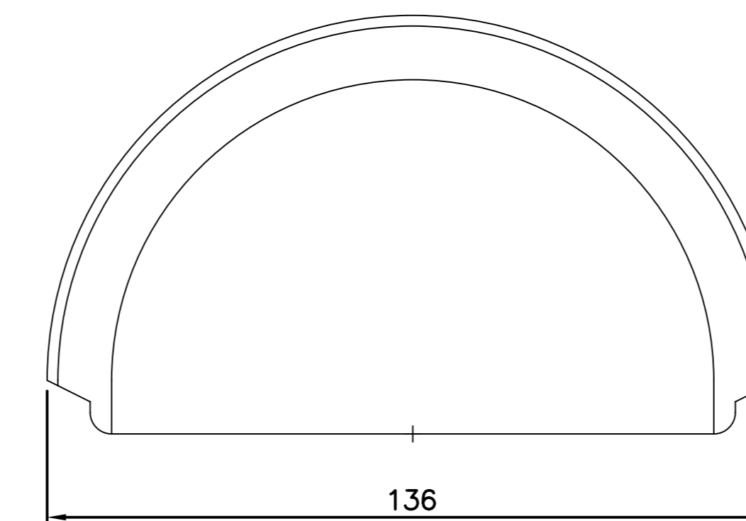
FG136 Zierstück
