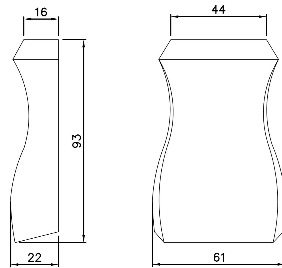
FG250 Zierstück
