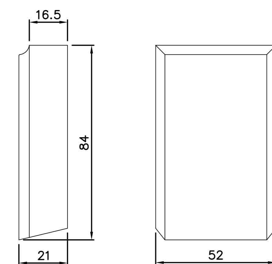
FG353 Zierstück
