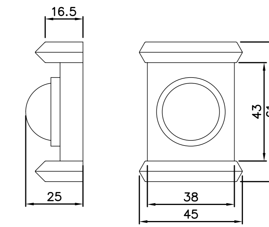
FG209 Zierstück
