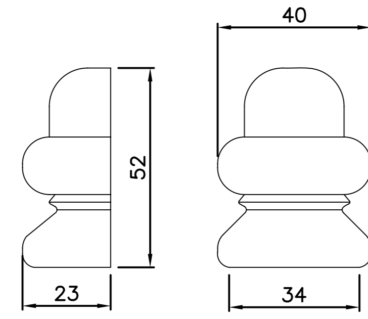
FG205 Zierstück
