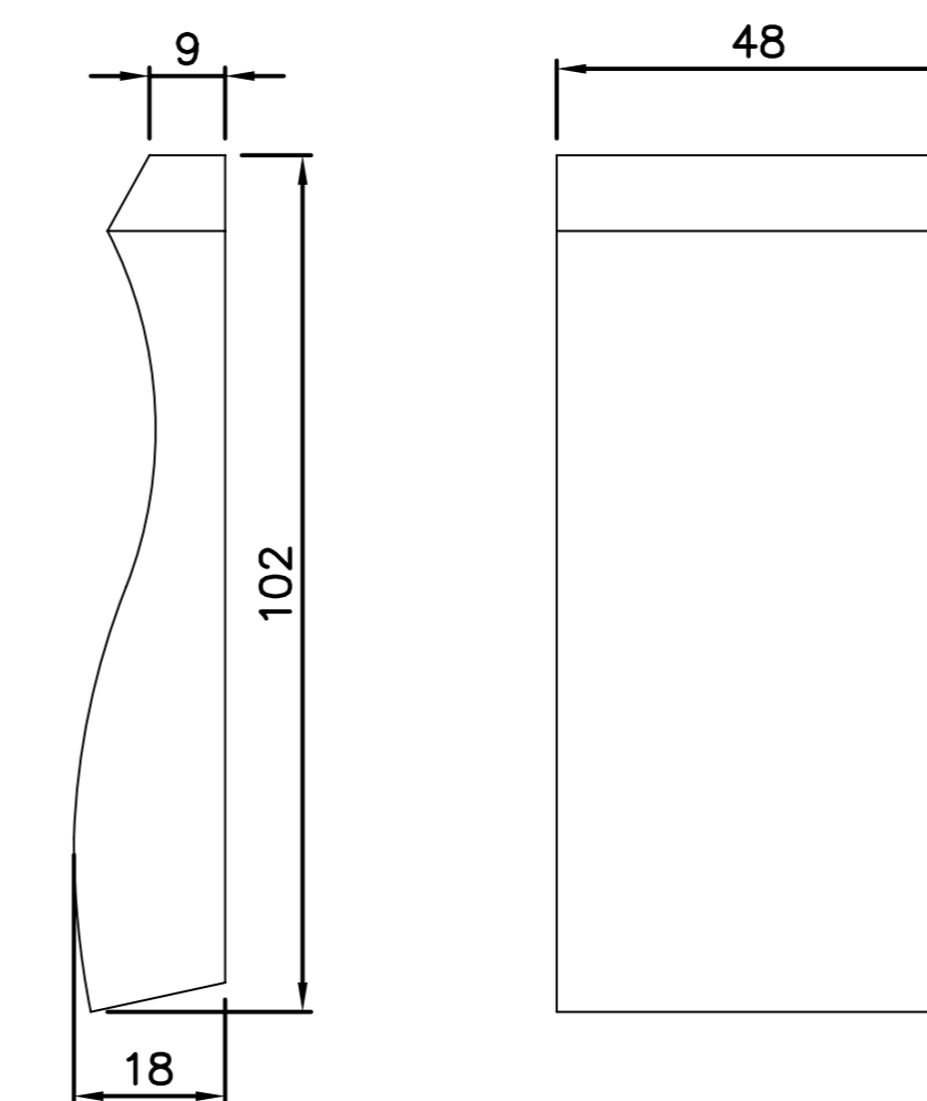
FG261 Zierstück
