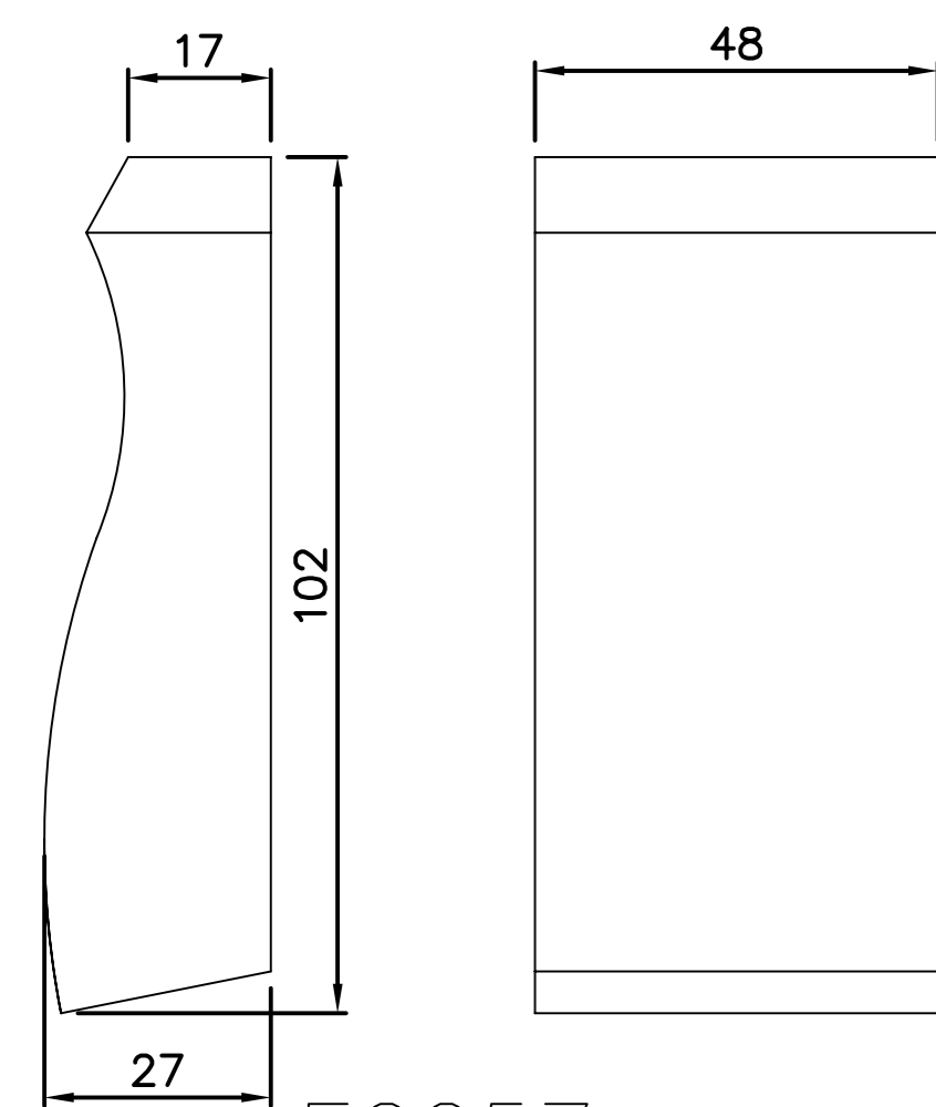
FG257 Zierstück
