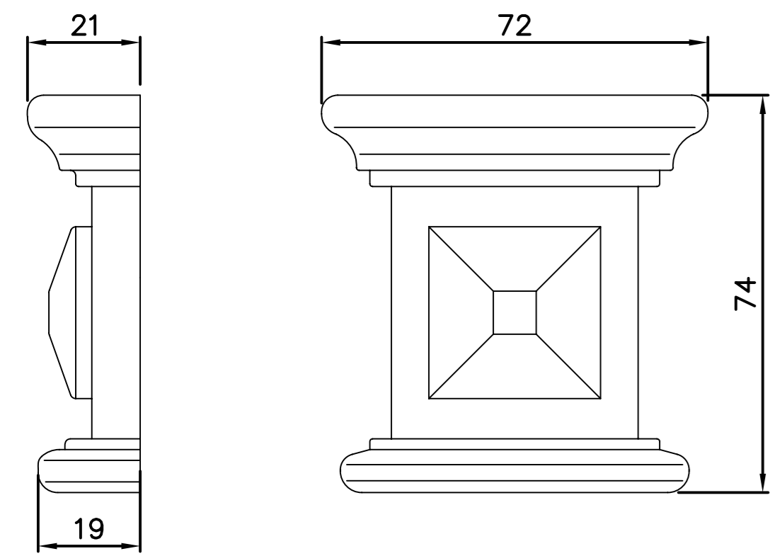
FG211 Zierstück
