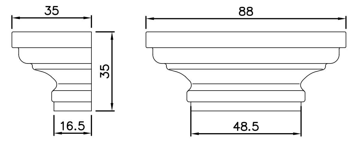
FG203 Zierstück
