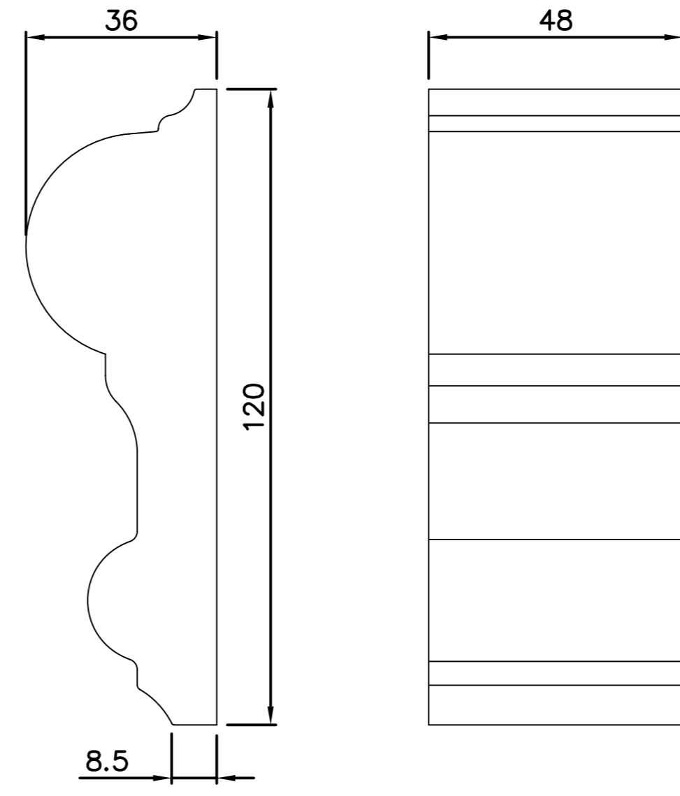
FG207 Zierstück
