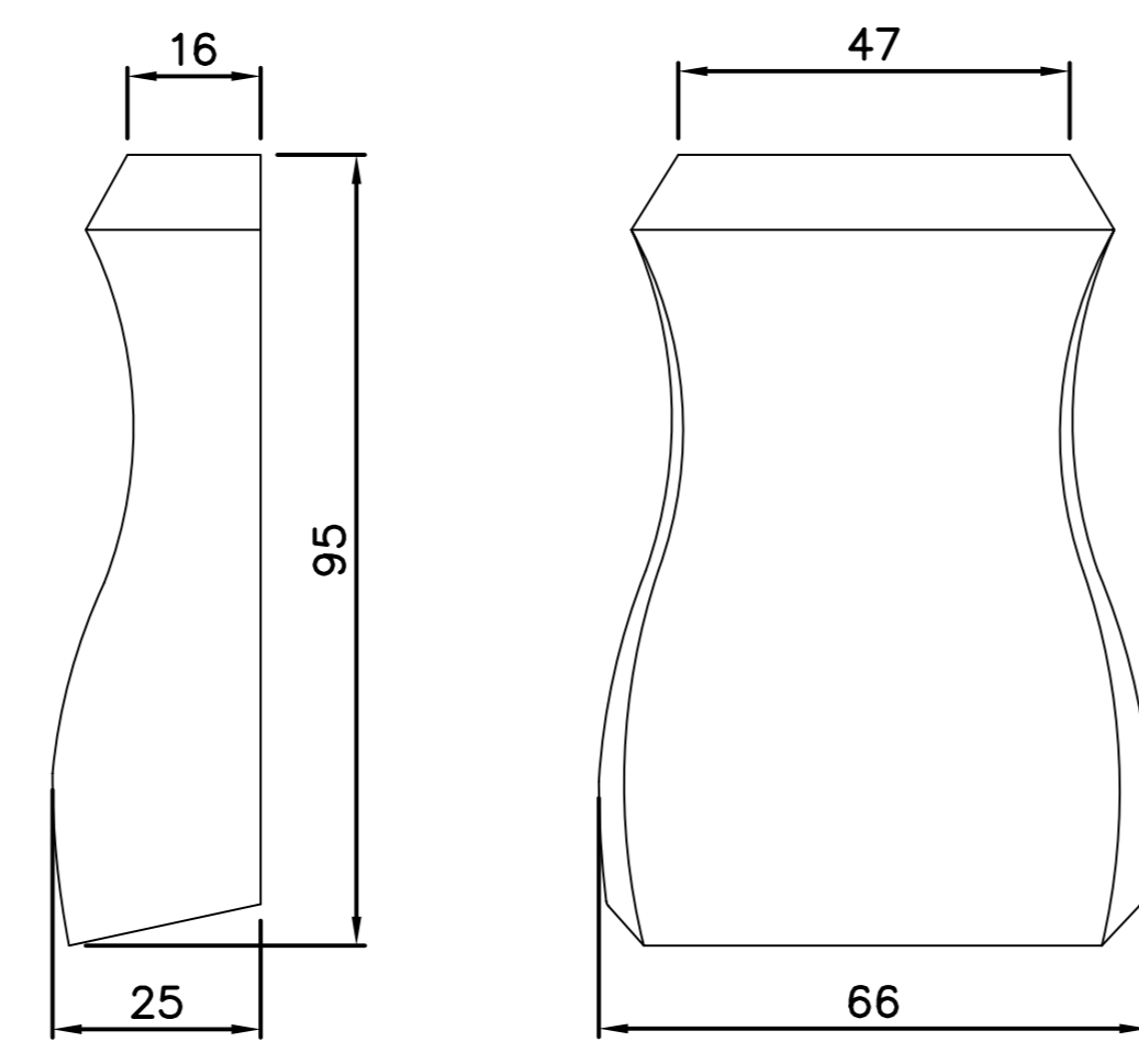
FG251 Zierstück
