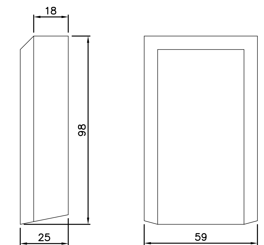
FG351 Zierstück
