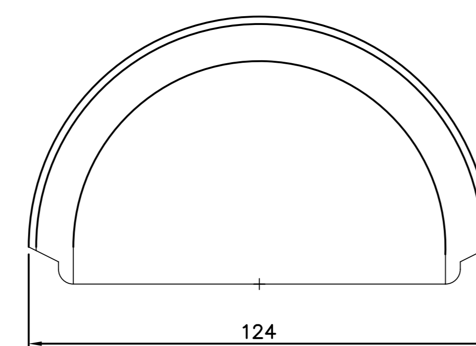
FG124 Zierstück
