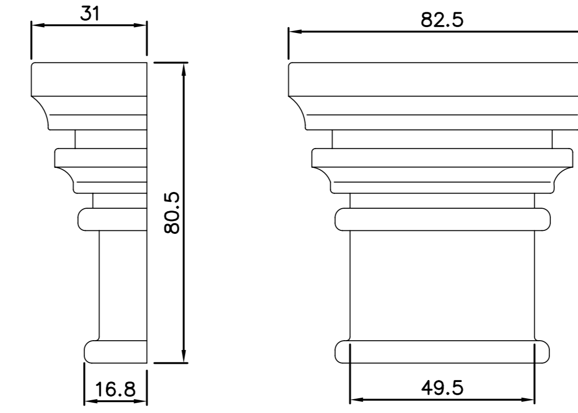
FG208 Zierstück
