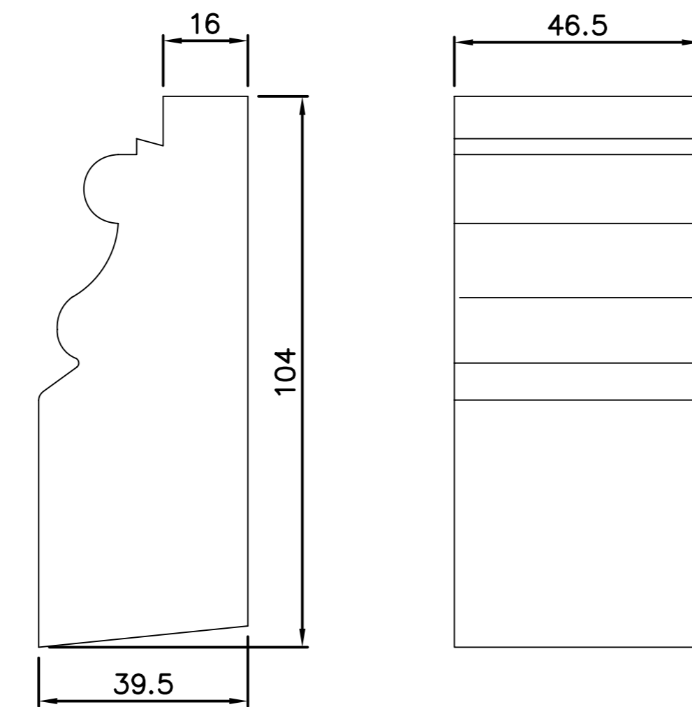
FG259 Zierstück
