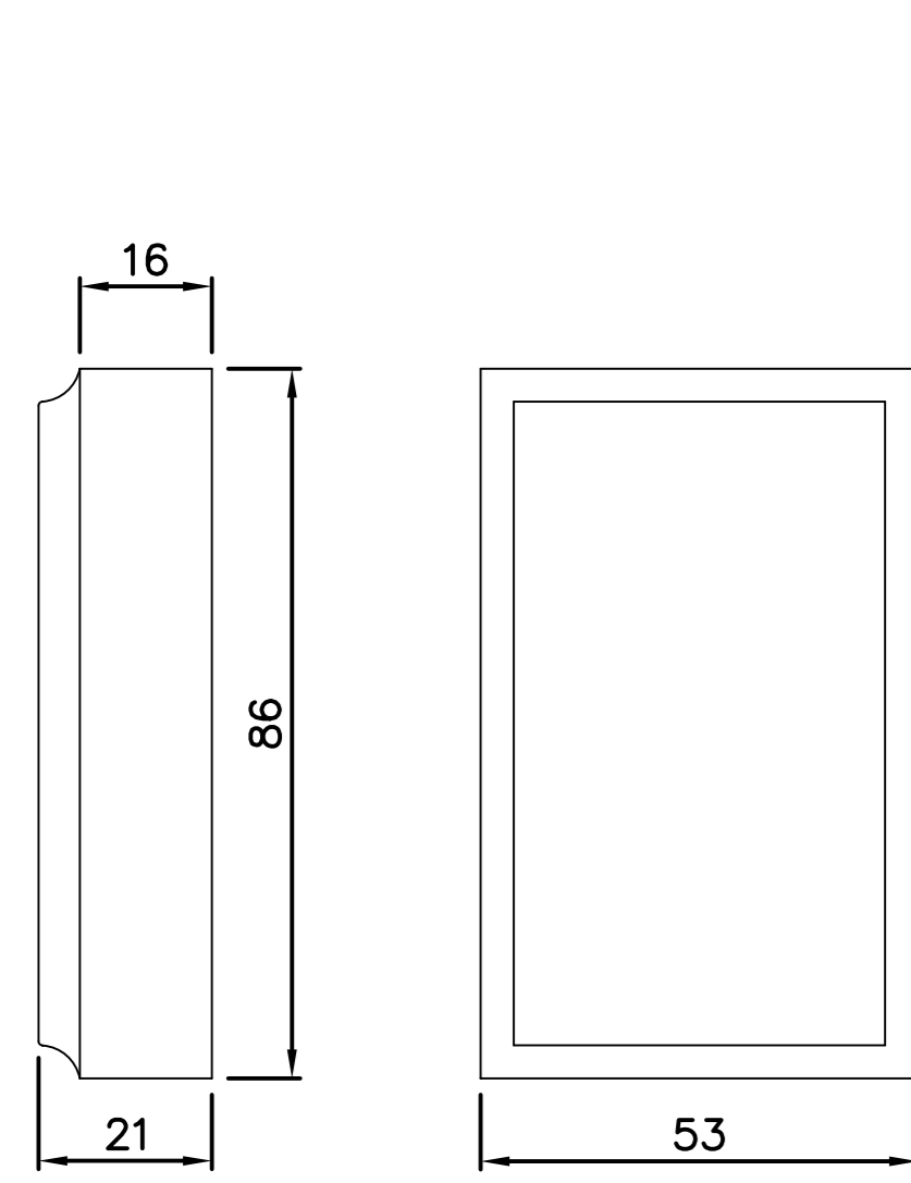
FG303 Zierstück
